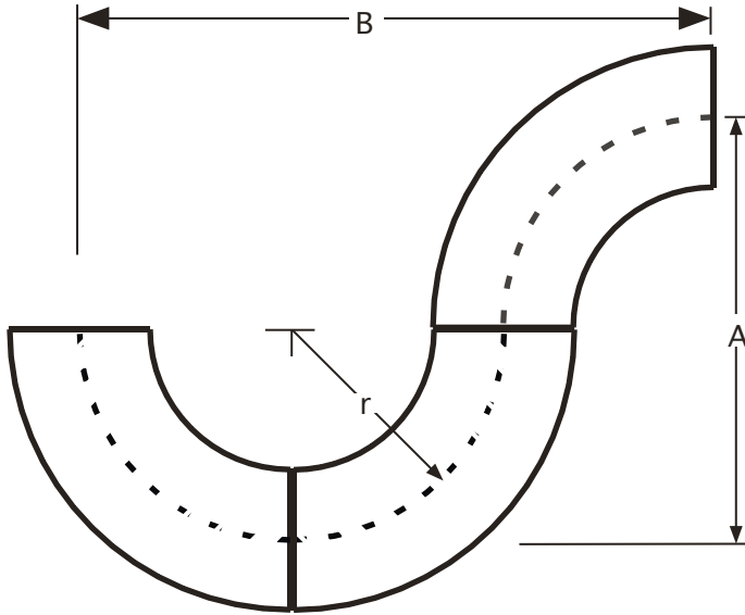
Long Radius P-Trap
