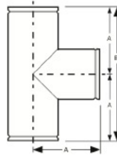
Roll grooved Tee
